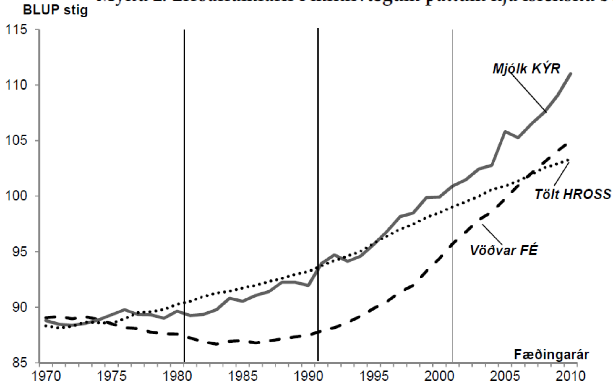
Mynd 2. Erfðaframarir í mikilvægum þáttum hjá íslensku búfé (ÁS 2012)
