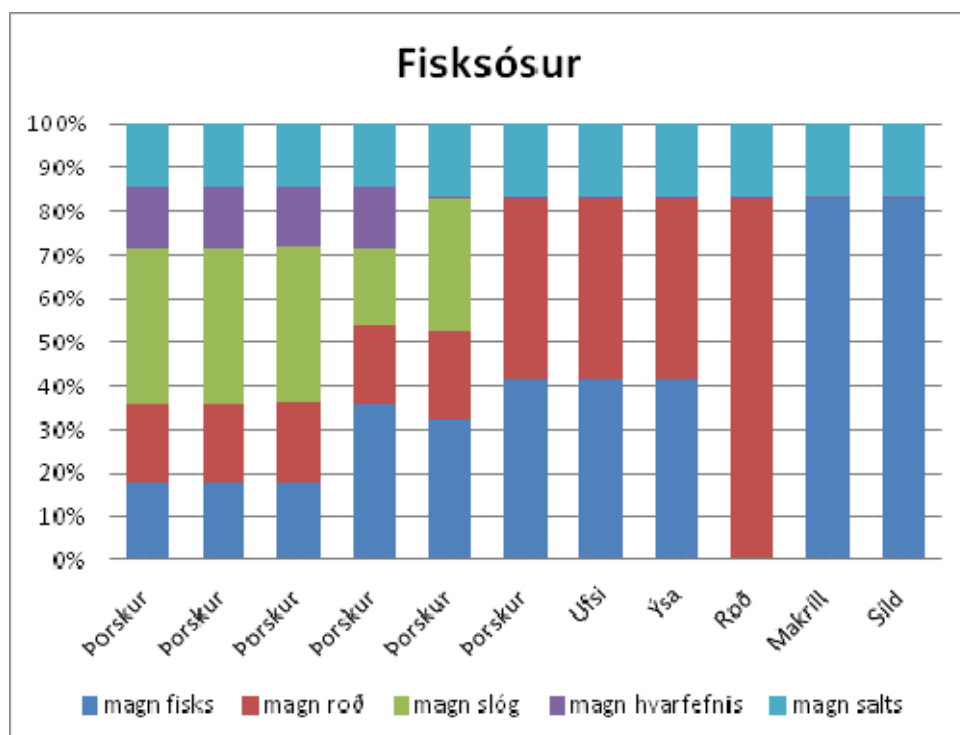
Mynd 3 Samsetning mauks til fisksósuframleiðslu á fyrstu stikum
